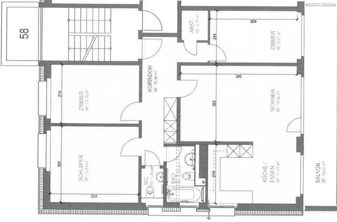
GRUNDRISS 1:100
